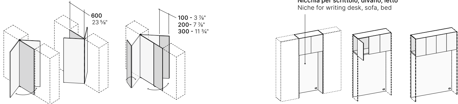
Apertura lato DX RH side opening
